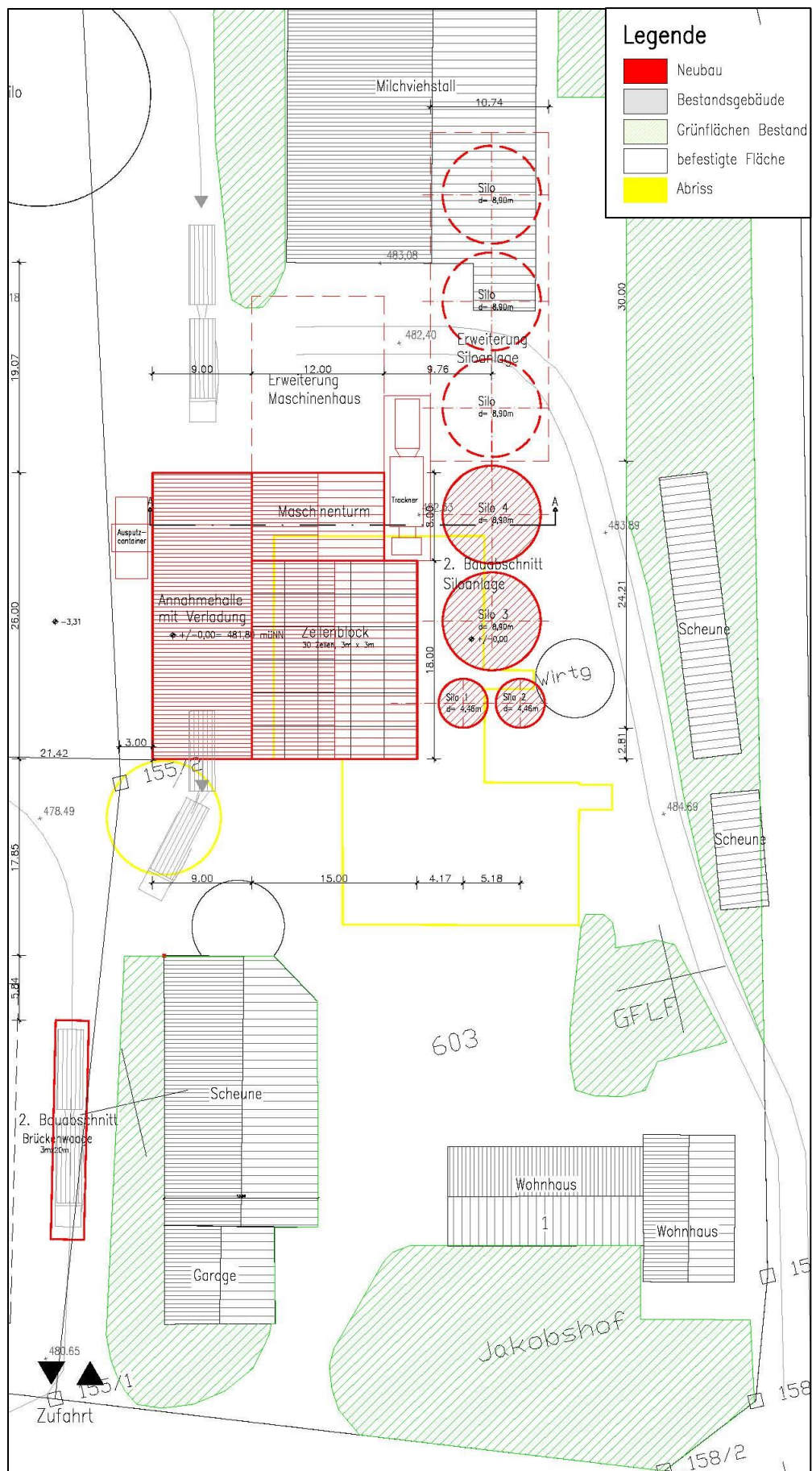
Abbildung 6: Entwurfsplan Neubau einer Getreideerfassungsanlage (HINTERLANG + BURK GMBH & CO. KG)
