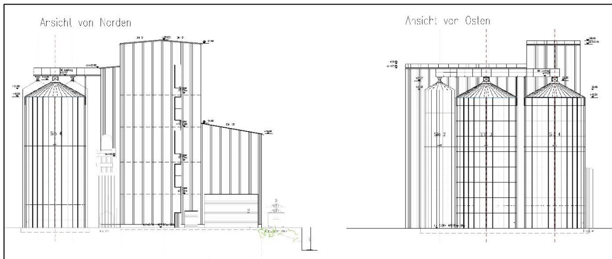
Abbildung 2: Getreideerfassungsanlage, Ansichten Norden/Osten (HINTERLANG + BURK GMBH & CO. KG)
